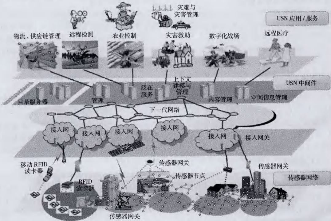
图 5 USN 体系框架
